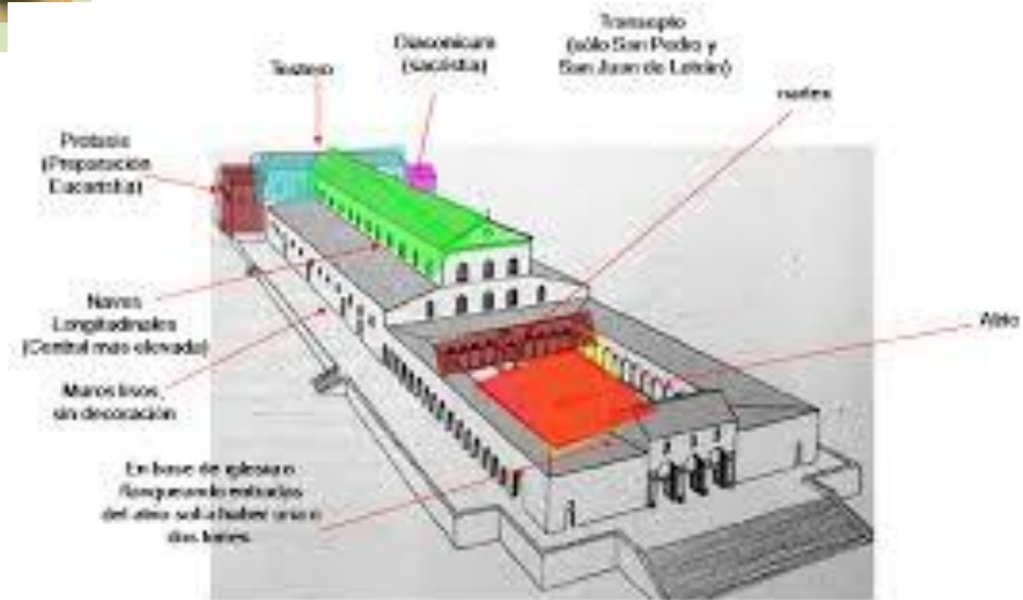
Pianta de Iglesias paleocristianas Primitiva basílica de San Pedro (reconstrucción)
