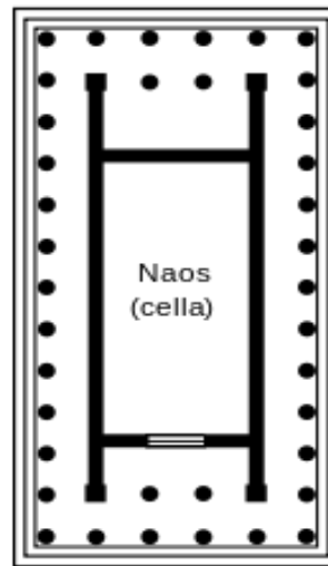
Períptero
