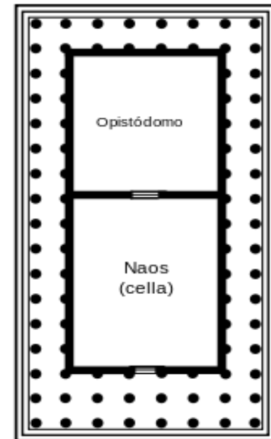
Pseudodíptero
