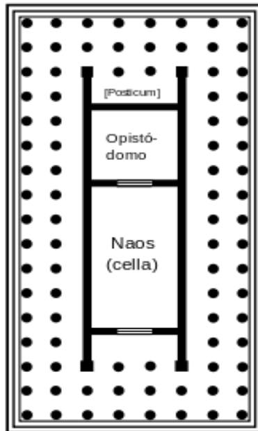
Díptero
